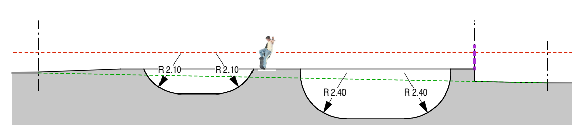
Schnitt 6- 6
