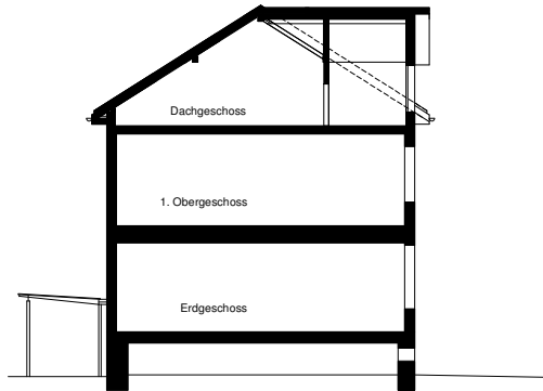
Schnitt A-A Bestand
