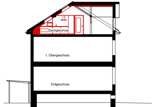
Schnitt A-A Projekt
